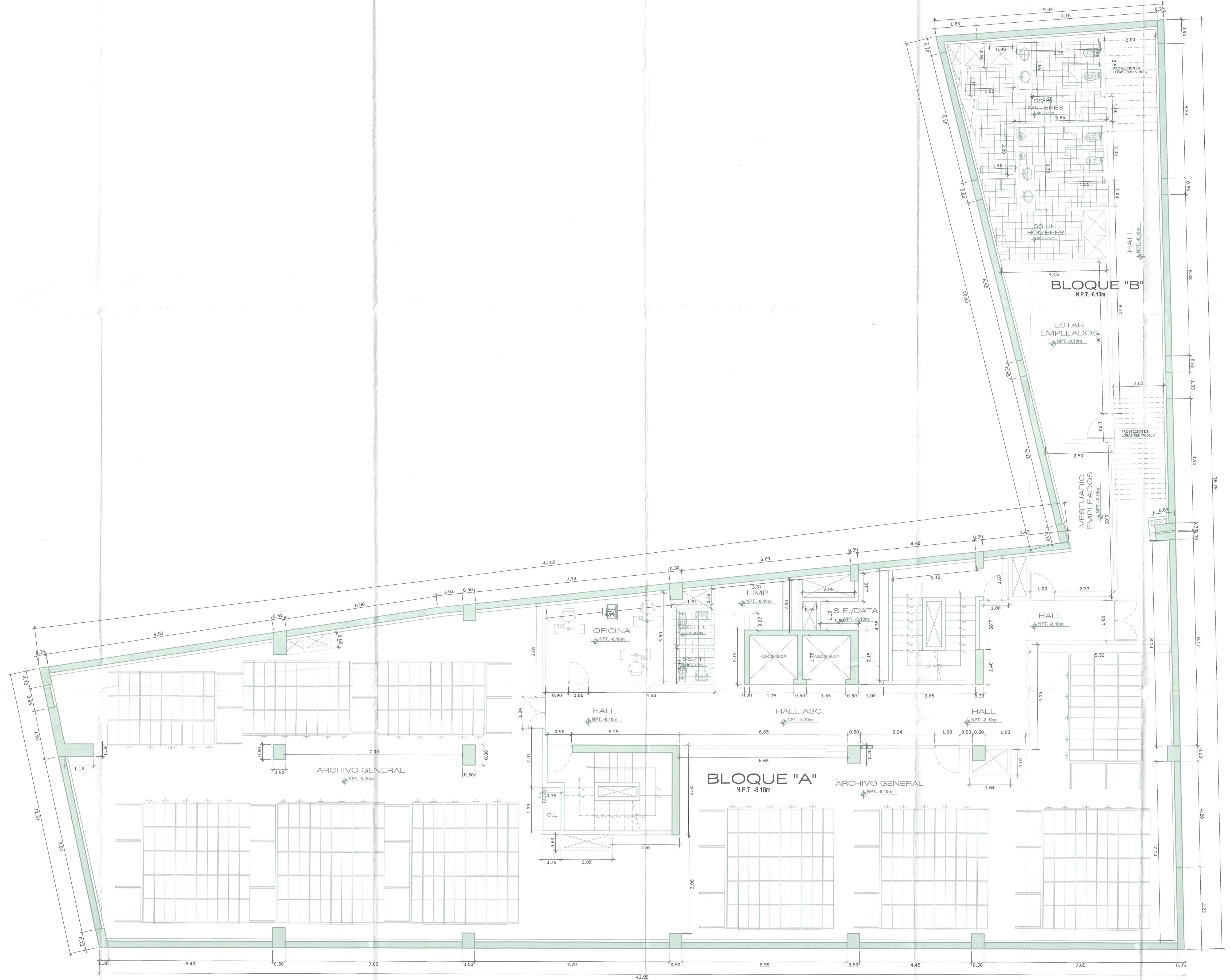
PLANTA DE DISTRIBUCIÓN ARQUITECTÓNICA - SÓTANO 02 ESCALA: 1:50
