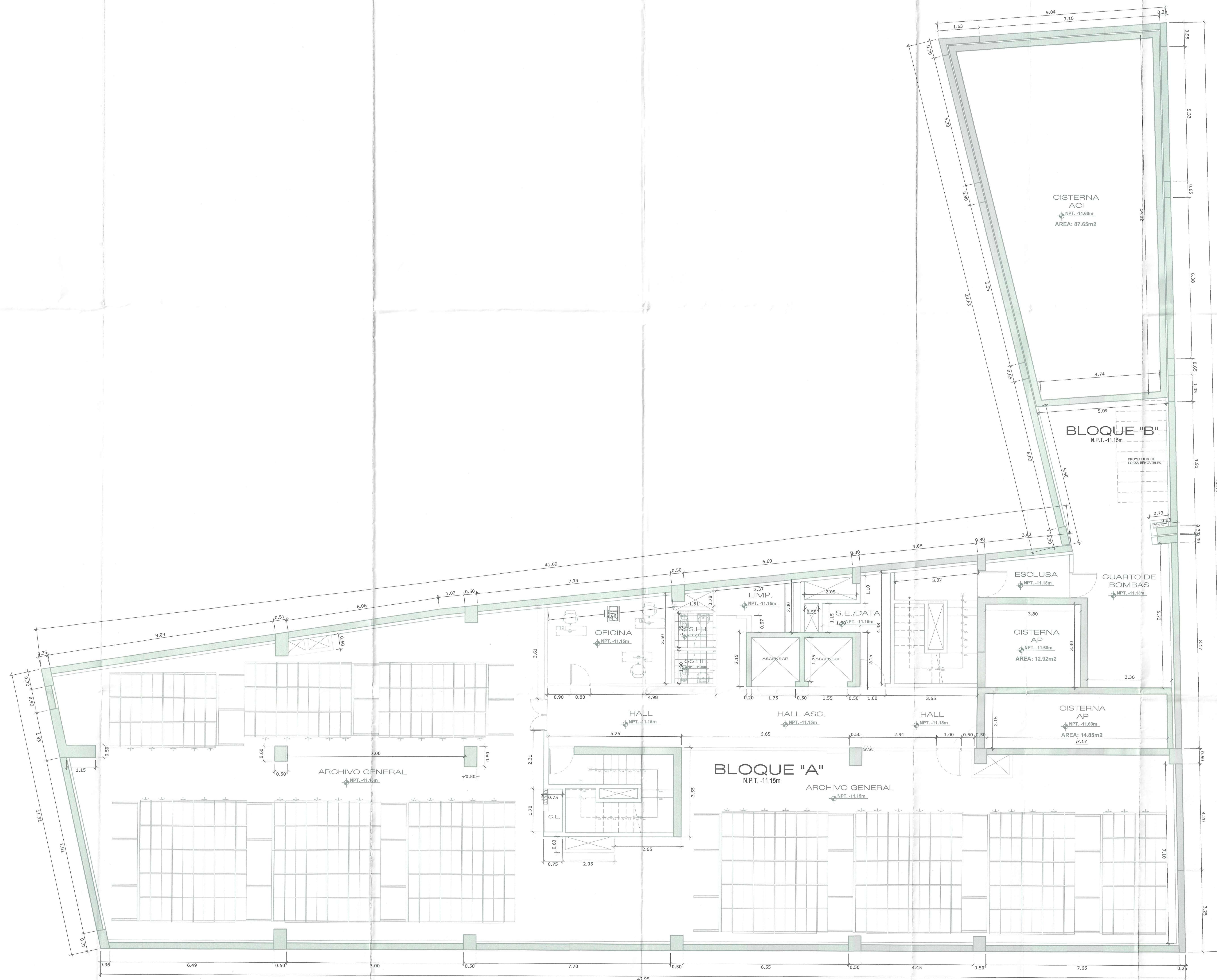
PLANTA DE DISTRIBUCIÓN ARQUITECTÓNICA - SÓTANO 03 ESCALA: 1:50
