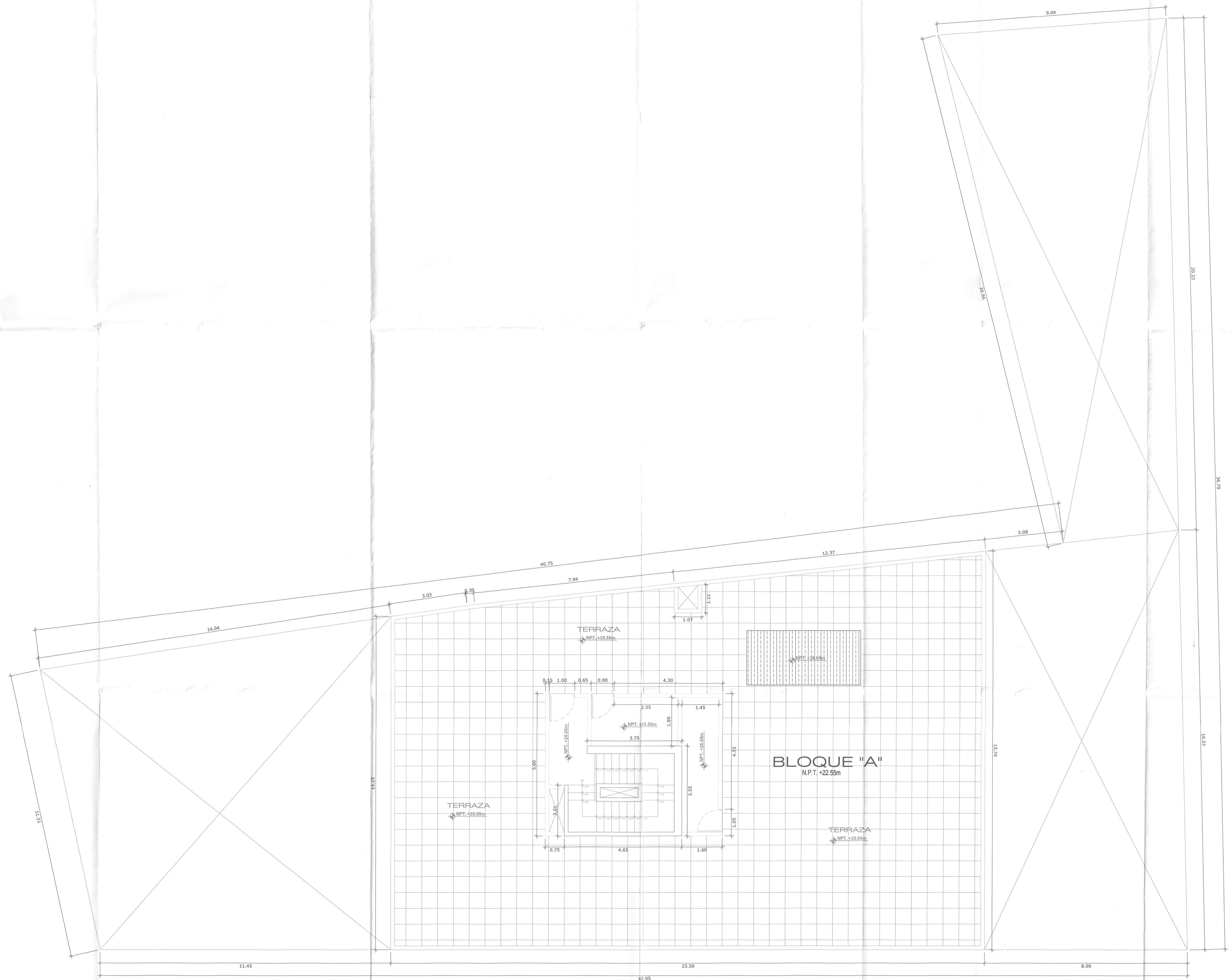
PLANTA DE DISTRIBUCIÓN ARQUITECTÓNICA - AZOTEA ESCALA: 1:50
