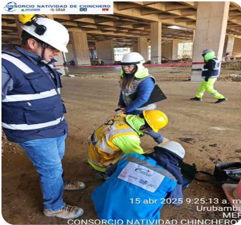
Medición de resistencia de pozos a tierra Measurements of resistance of grounded wells
