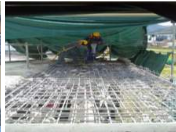
d) DEMOLICIÓN DE LOSA DEFLECTADA – ADICIONAL N°05
