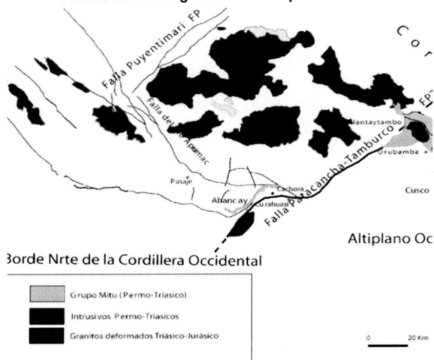
Gráfico 02: Geología de Usnomoqo- Tamburco
